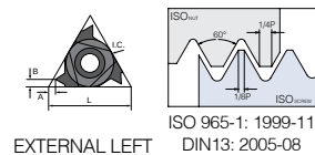
EXTERNAL LEFT ISO 965-1: 1999-11 DIN13: 2005-08
