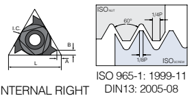
INTERNAL RIGHT ISO 965-1: 1999-11 DIN13: 2005-08
