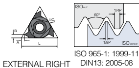
EXTERNAL RIGHT ISO 965-1: 1999-11 DIN13: 2005-08
